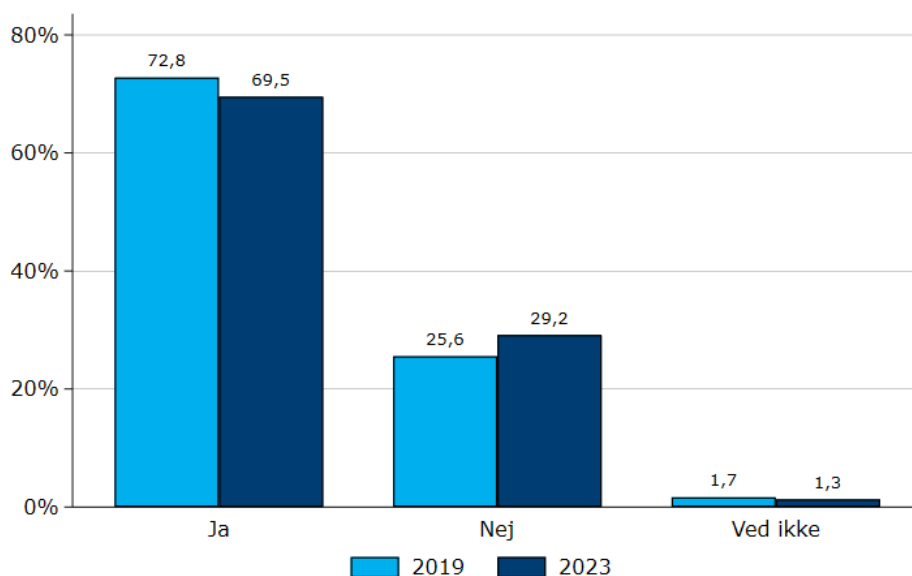
Figur 5. Borgmesterkoalition
